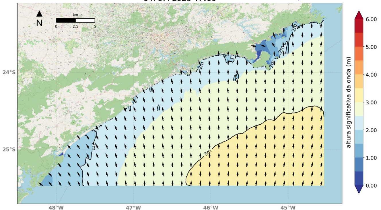
Figura 3. Resultado do modelo de ondas para o litoral de São Paulo durante sábado (04/07) às 17h. A escala de cores representa a altura significativa das ondas (m).
